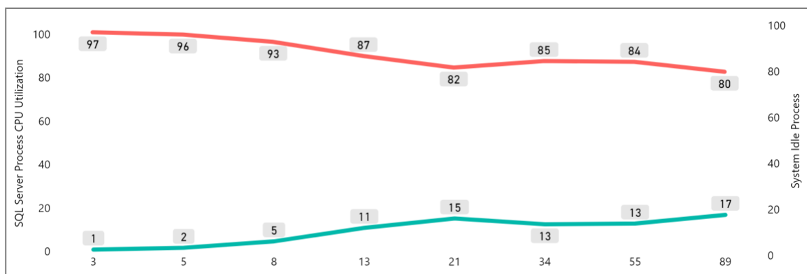
Figure 15 – SQL Server 2008 R2 avec 16 vCores : durée d'utilisation de l'unité centrale par rapport à la durée de veille sous forme de pourcentage
