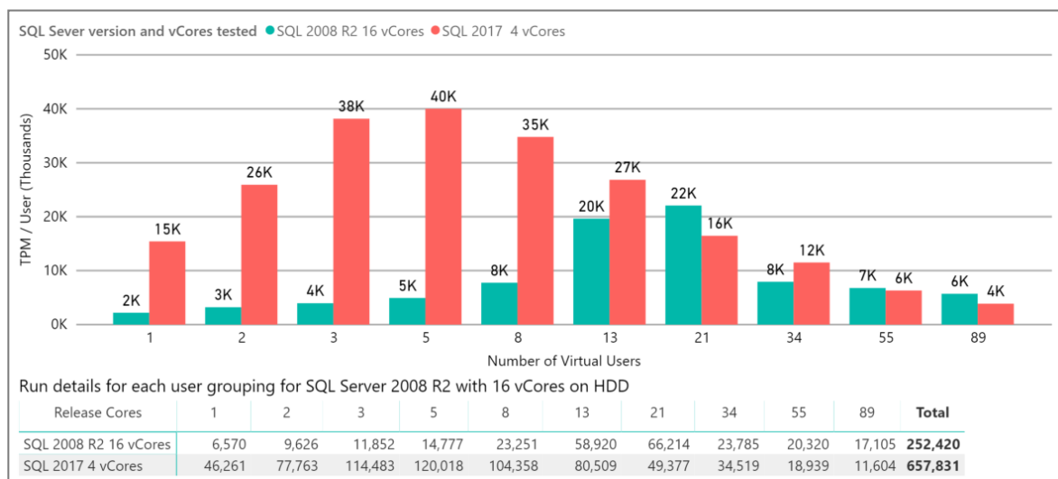
Figure 18 – Comparaison TPM / Utilisateur pour SQL Server 2017 R2 avec 4 vCores et SQL Server 2008 R2 avec 16 vCores
