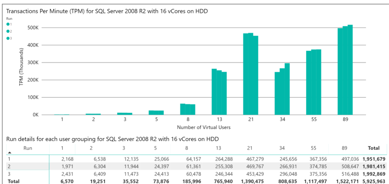
Figure 11 – Résultats de SQL Server 2008 R2 avec 16 vCores sur disques durs
