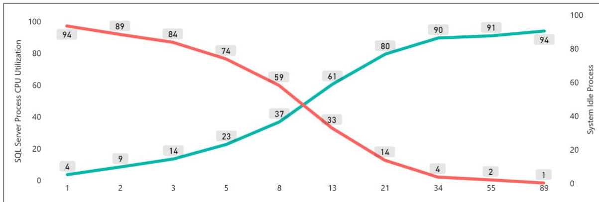
Figure 14 – SQL Server 2017 avec 8 vCores : durée d'utilisation de l'unité centrale par rapport à la durée de veille sous forme de pourcentage
