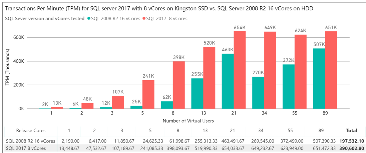
Figure 16 – Comparaison entre SQL Server 2008 R2 avec 16 vCores et SQL Server 2017 avec seulement 8 vCores
