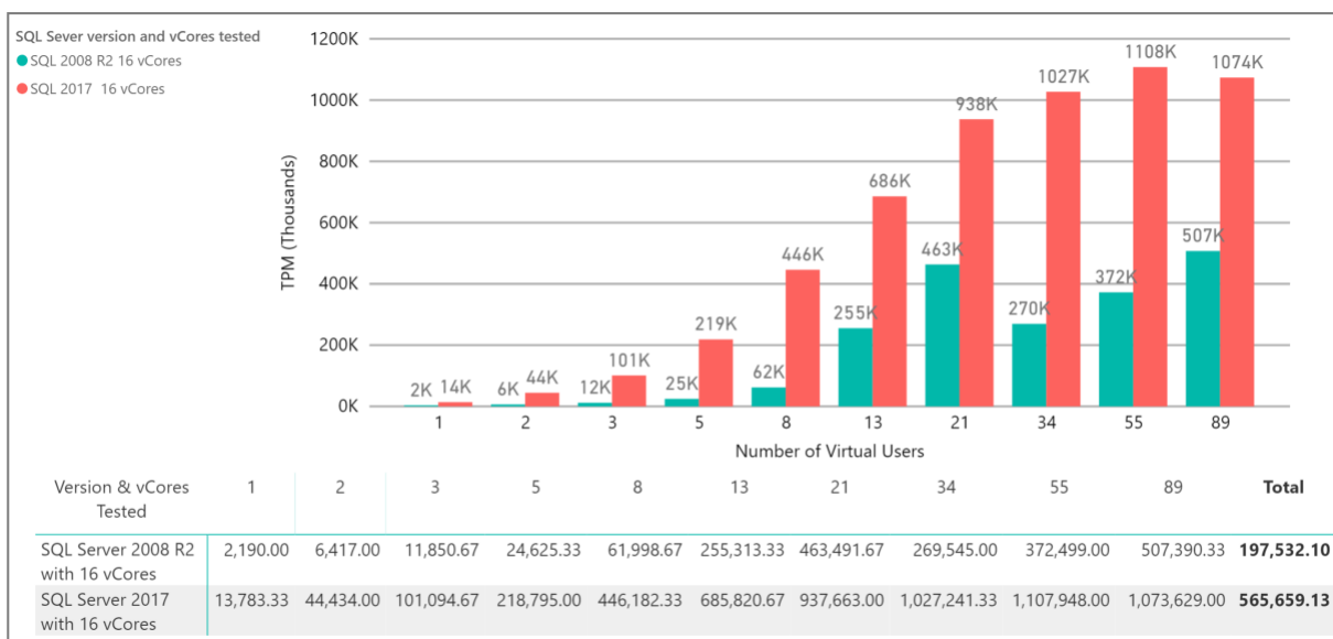
Figure 13 – Comparaison entre SQL Server 2008 R2 sur disques durs et SQL Server 2017 sur SSD DC500M avec 16 vCores
